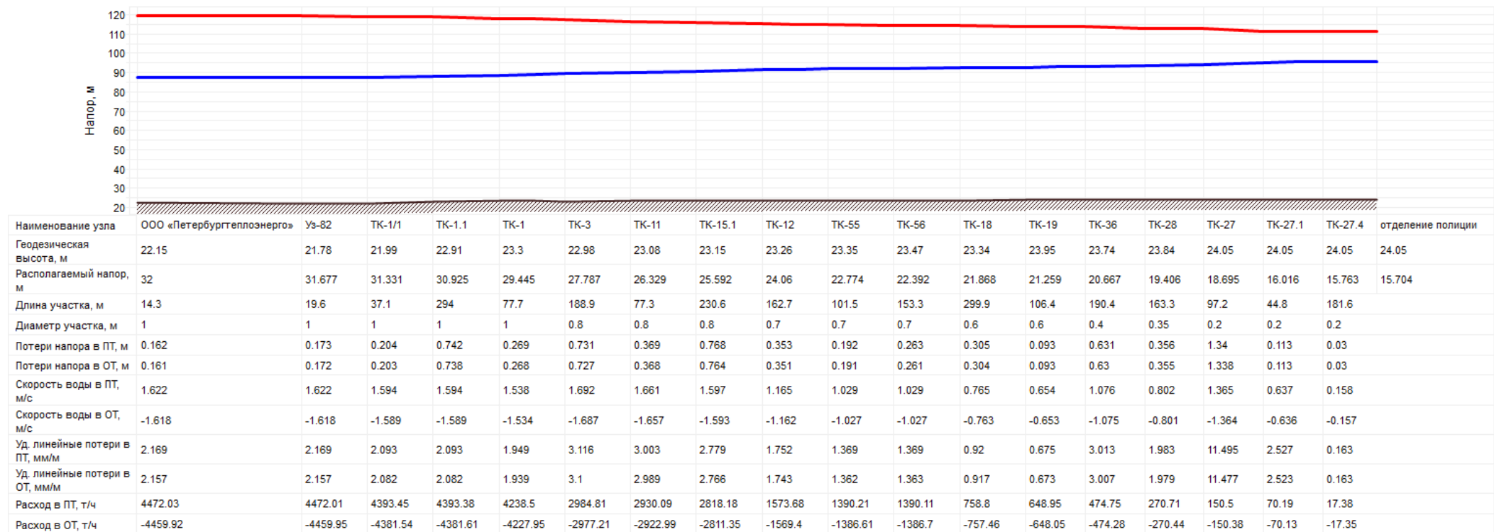
Рисунок 26. Пьезометрический график участка тепловой сети от котельной ООО «Петербургтеплоэнерго» до перспективного потребителя Отделение полиции
