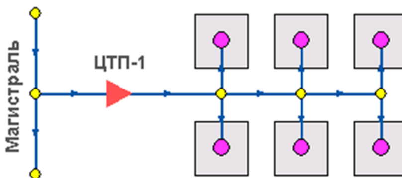
Рисунок 5. Изображение ЦТП
