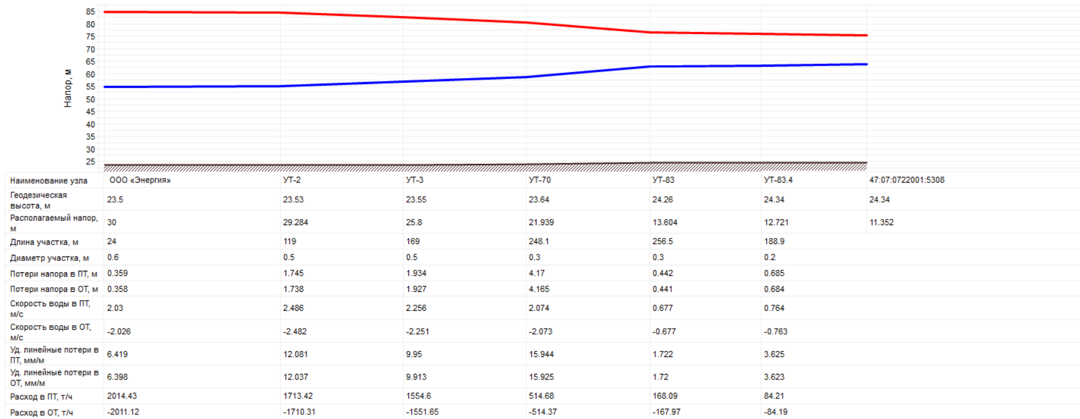
Рисунок 28. Пьезометрический график участка тепловой сети от котельной ООО «Энергия» до перспективного потребителя
